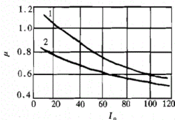
图 10.1 修正系数 \mu
