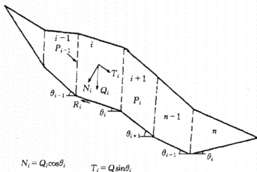
图 5.1 滑坡稳定系数计算
