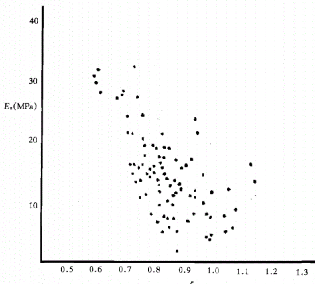
图 3.2 压缩模量与孔隙比的散点图
