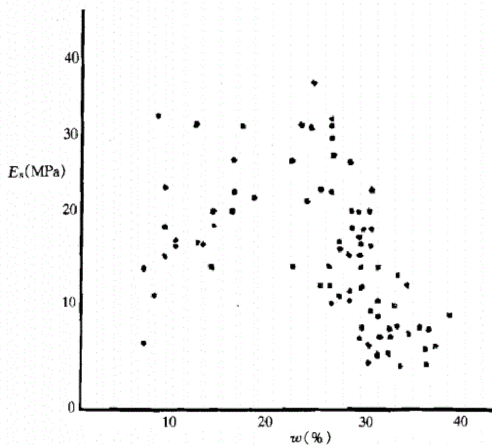
图 3.3 压缩模量与含水量的散点图
