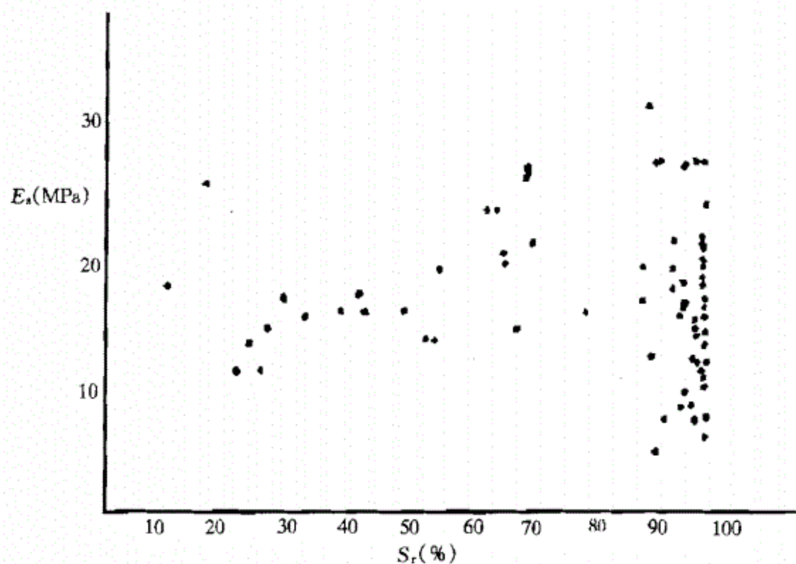
图 3.4 压缩模量与饱和度的散点图
