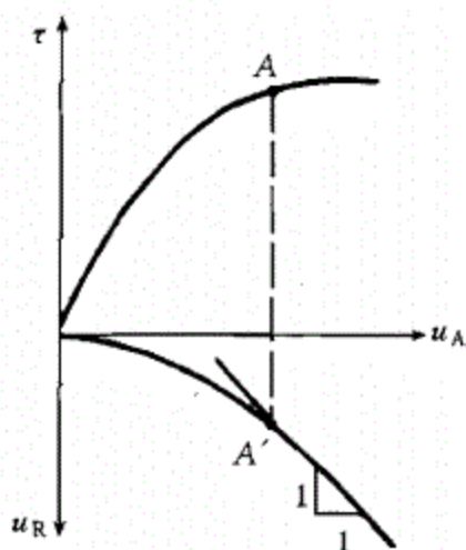
图 10.3 确定屈服强度的辅助方法
