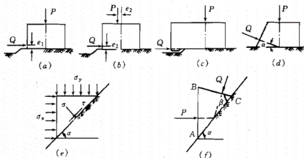
图 10.2 现场直剪方案布置
