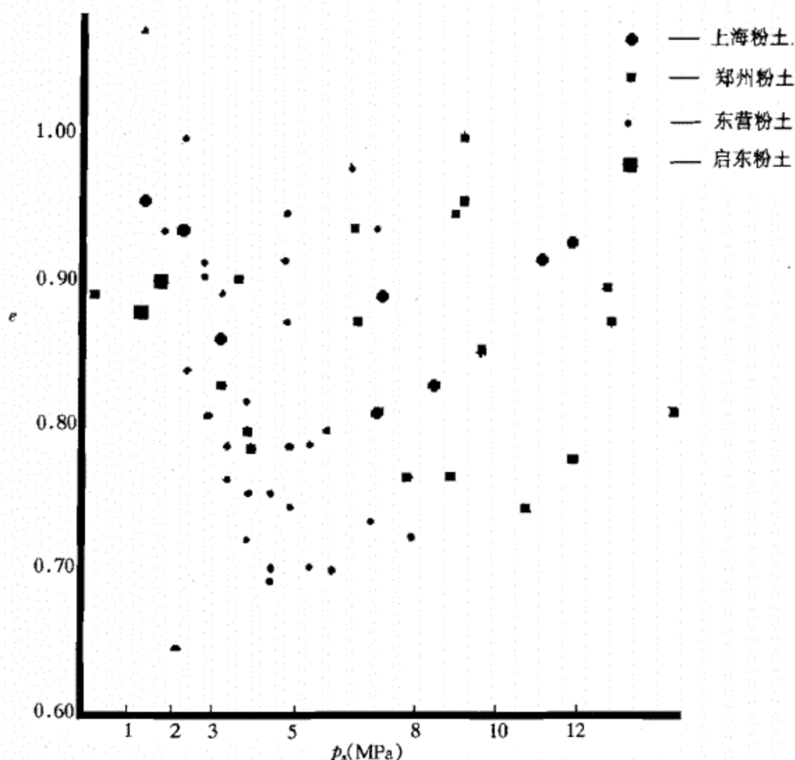
图 3.1 孔隙比与比贯入阻力的散点图
