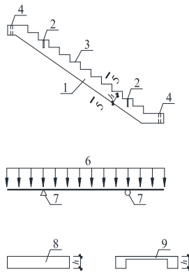
图 3 装配式混凝土楼梯吊装计算简图
