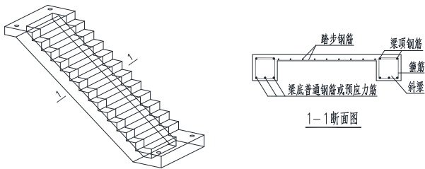
图2 预制梁式楼梯示意
