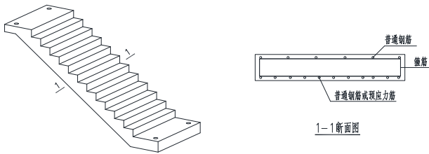
图1 预制板式楼梯示意
