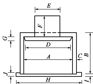
图 A.1 压碎值试模
