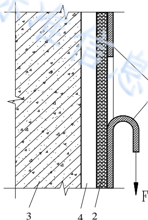
图 7.1.3 密封胶现场剥离法检测示意图
