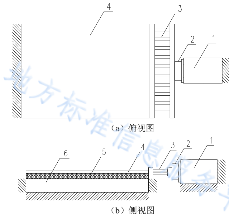
图 4.4.4 多个拉结件的群锚整体抗剪承载力检测加载示意图
