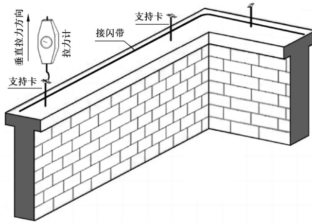
图 B.3 卡夹器连接固定支架(可拆卸)垂直拉力测量示意图
