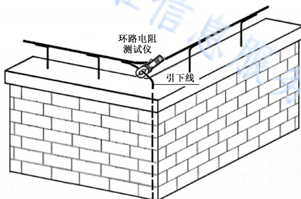
图 C.2 防雷引下线贯通性判定
