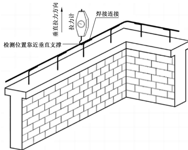
图 B.1 焊接方式连接固定支架垂直拉力测量示意图
