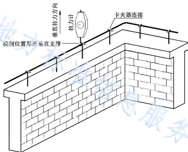
图 B.2 卡夹器连接固定支架(无法拆卸)垂直拉力测量示意图
