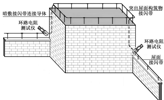
图 C.3 不等高暗敷接闪带闭合性判定
