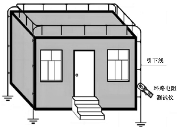
图 C.1 防雷引下线环路电阻(近似等于接地电阻)测量
