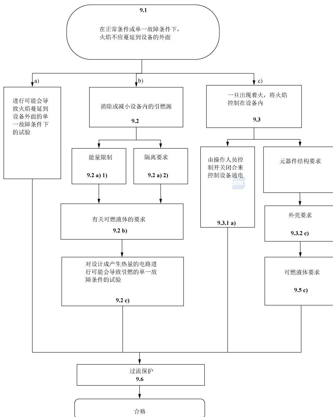
图 7 防止火焰蔓延要求的流程图
